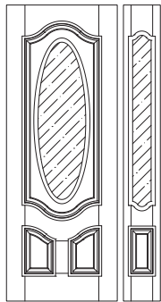
GP132 Door and Sidelite
