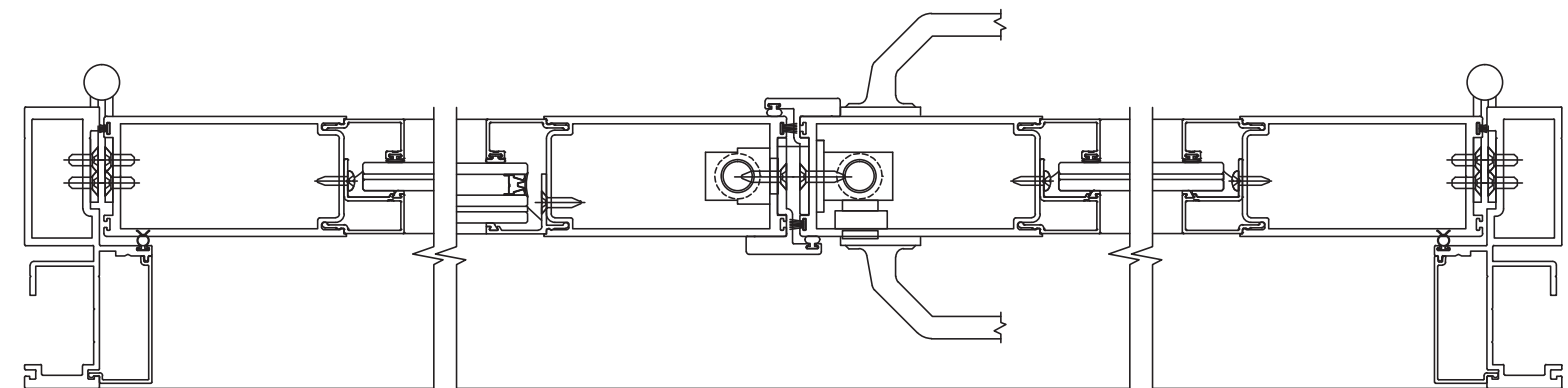
STANDARD DOOR FRAMES INSWING
